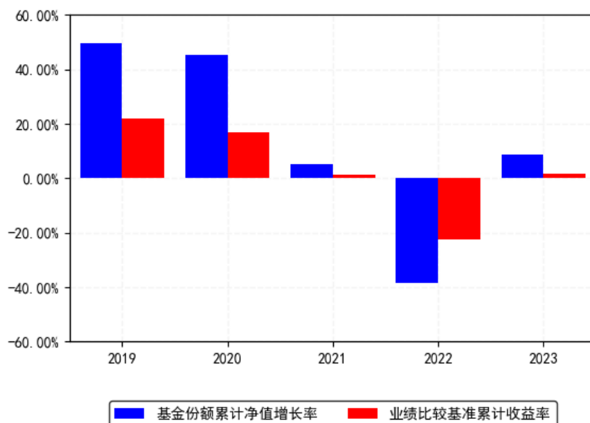
南方信息创新混合C每年净值增长率与同期业绩比较基准收益率的对比图（2023年12月31日）
